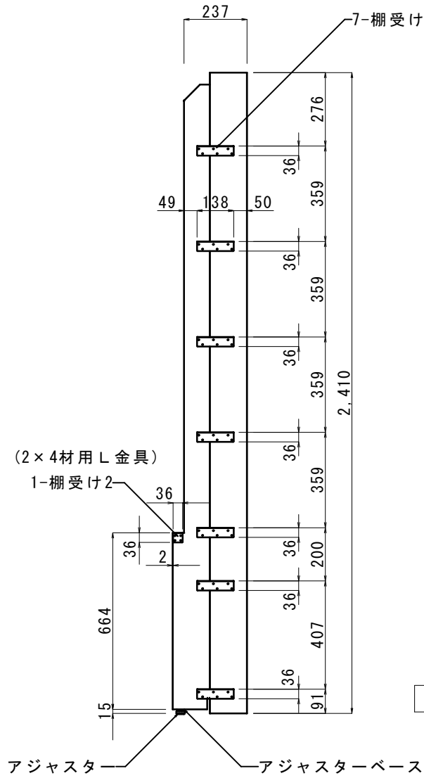
右側面図
